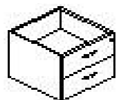
CAJONERA FLOTANTE 41 X 50 PROF. X 27 ALT.
