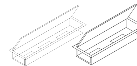
PASACABLE SIMPLE: 27,5 X 11X5 PASACABLE DOBLE: 42,5 X 11,5
